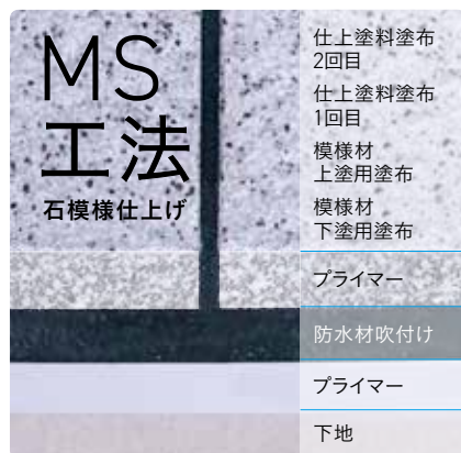
工程見本：MS工法（石模様仕上げ）
